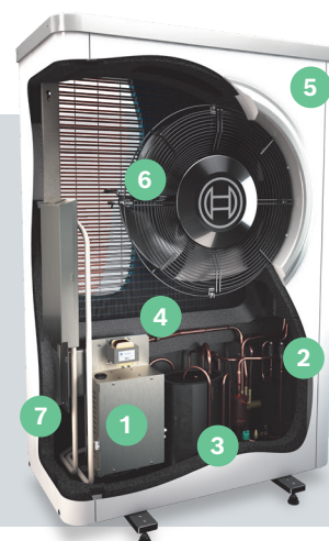
Außenaufstellung Compress 7000i AW OR
