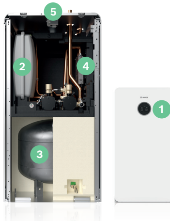
Der „Plug & Play“-Puffertower Sanierungsoptimiert bei flexiblem Warmwasser-Komfort
